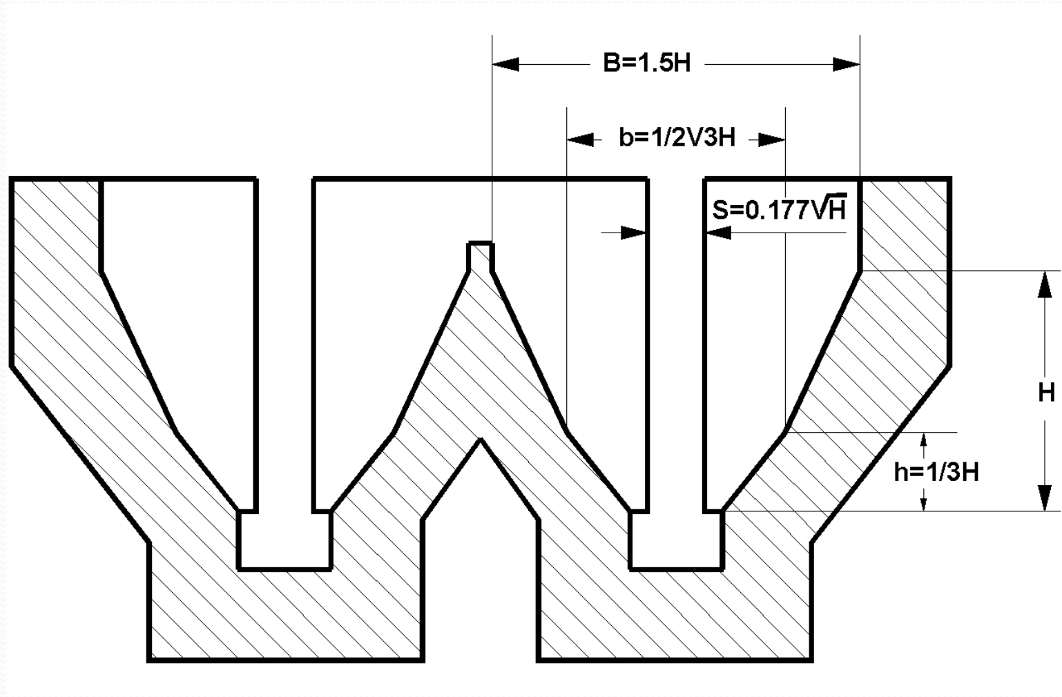
Section hexagonale d'un dessableur à section parabolique.
