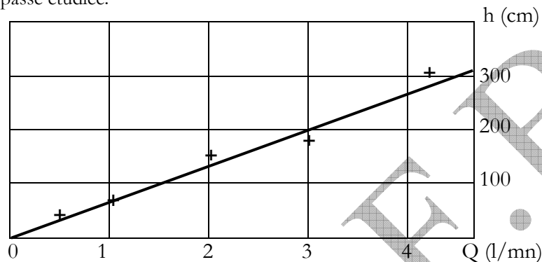
Figure 6.2 : Graphique hauteur-débit pour un essai à niveau constant
